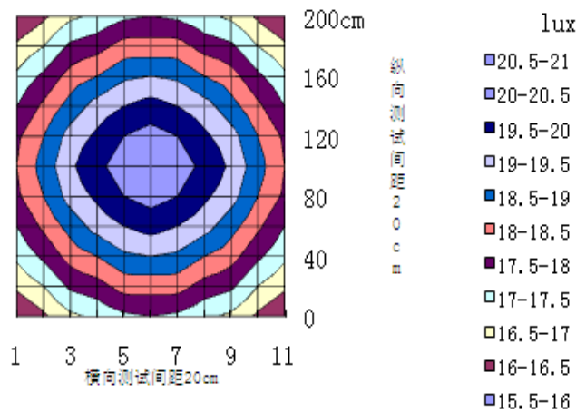
7W LED灯泡照度图 (2.5m)
