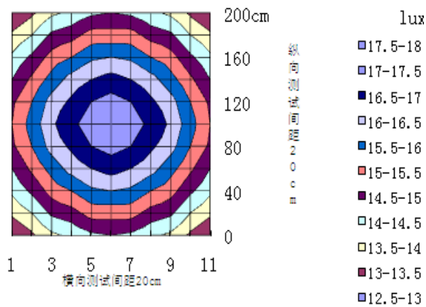
6W LED灯泡照度图 (2.5m)
