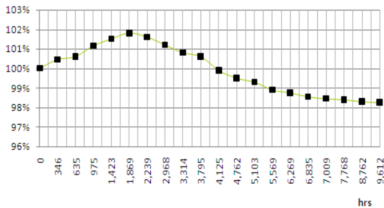
灯泡光衰曲线图
