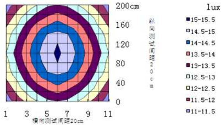
5W LED灯泡照度图 (2.5m)
