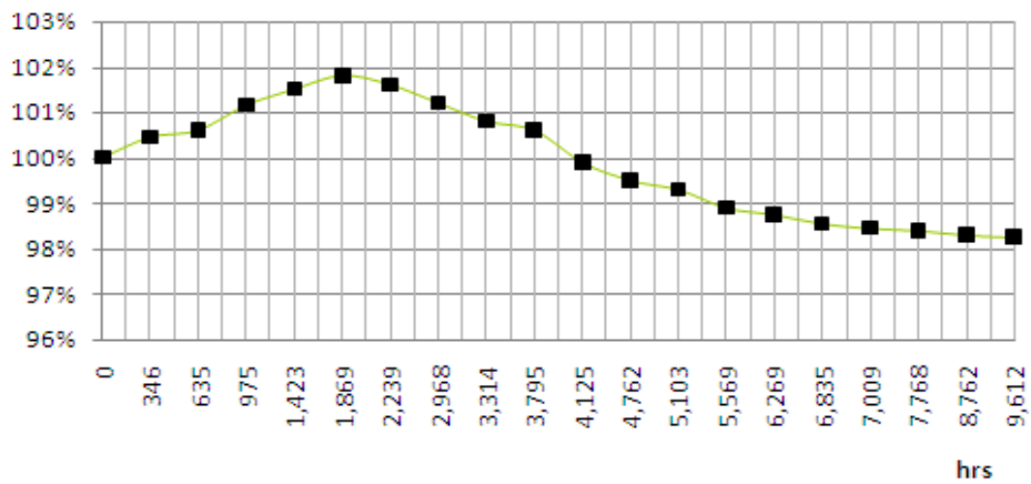
灯泡光衰曲线图
